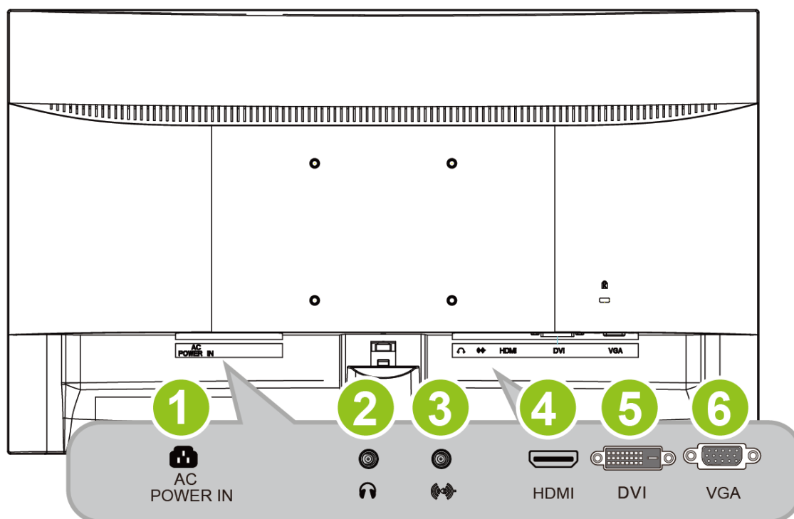
Figura 2. Branchement à un pc
