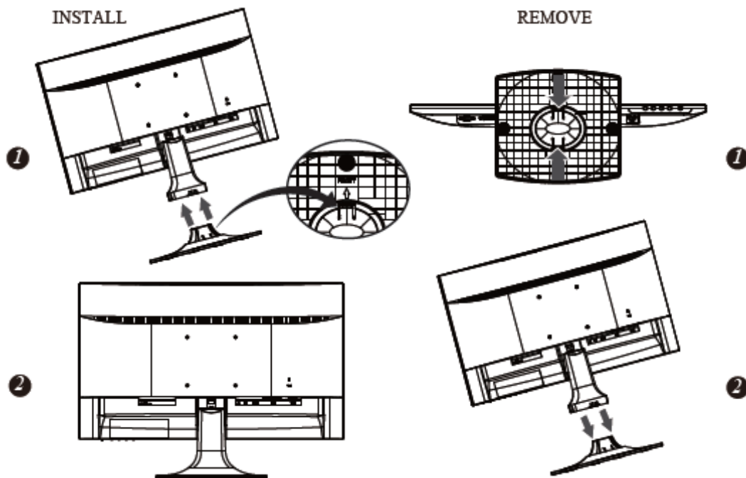
Figure.1. Installer et enlever l'embase
